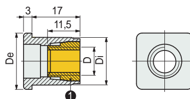
Dimensiones tubo
