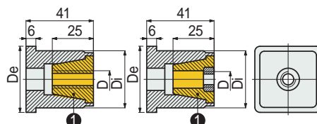
Cono de expansión de latón
