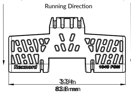
Vista superior de cadena con superficie abierta FG (35% abierta)
