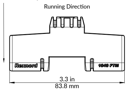
Vista superior de cadena con superficie cerrada FT
