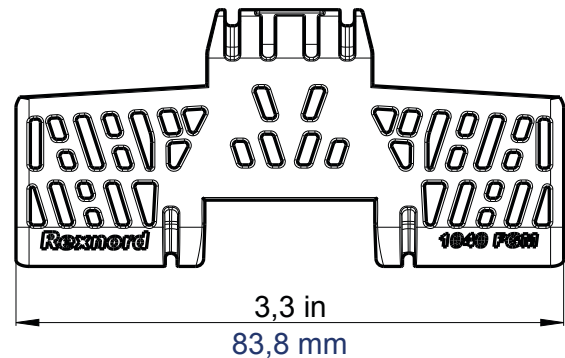
Vista superior de la banda modular (35 % de área abierta)
